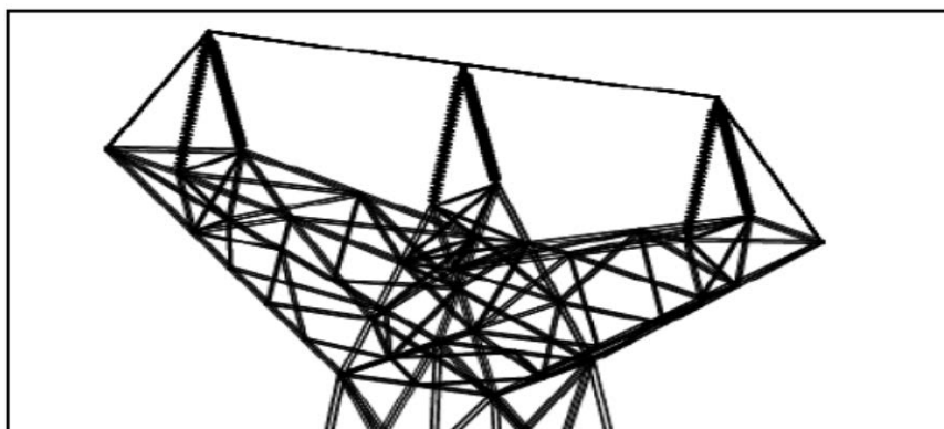
Рис.5. Проект установки на траверсах опор решетчатого типа опорных композитных изоляторов повышенной прочности для изолированного крепления проводов
