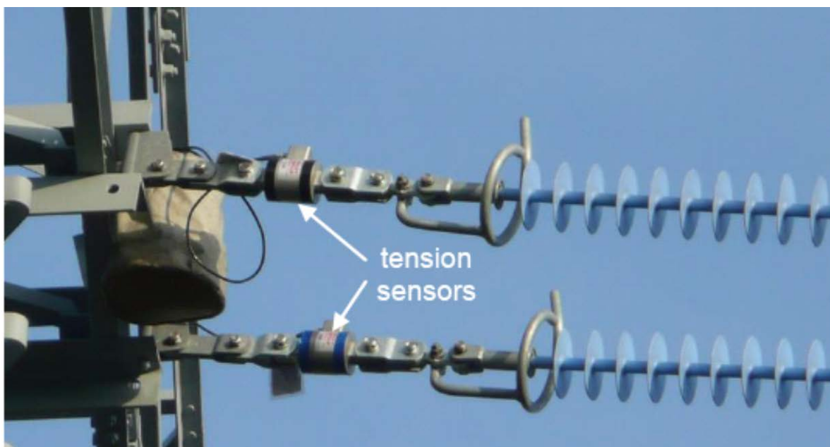
Рис. 16. Датчики для измерения тяжения проводов ВЛ 220 кВ
