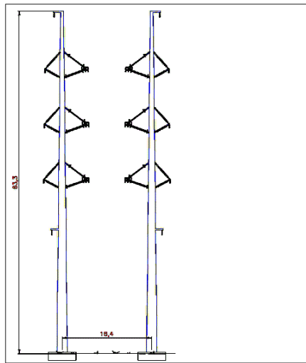
Рис.12. Опора из двух стоек и опорные изоляторы с шарнирным креплением для подвески проводов расщеплённых фаз
