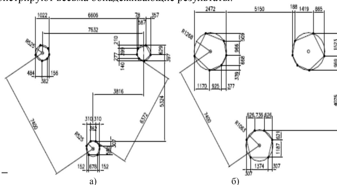
Рис.13. Ассиметричная форма расщеплённых фаз а- уменьшение размеров пучка проводов у опор. б- увеличение размеров пучка в середине пролёта
