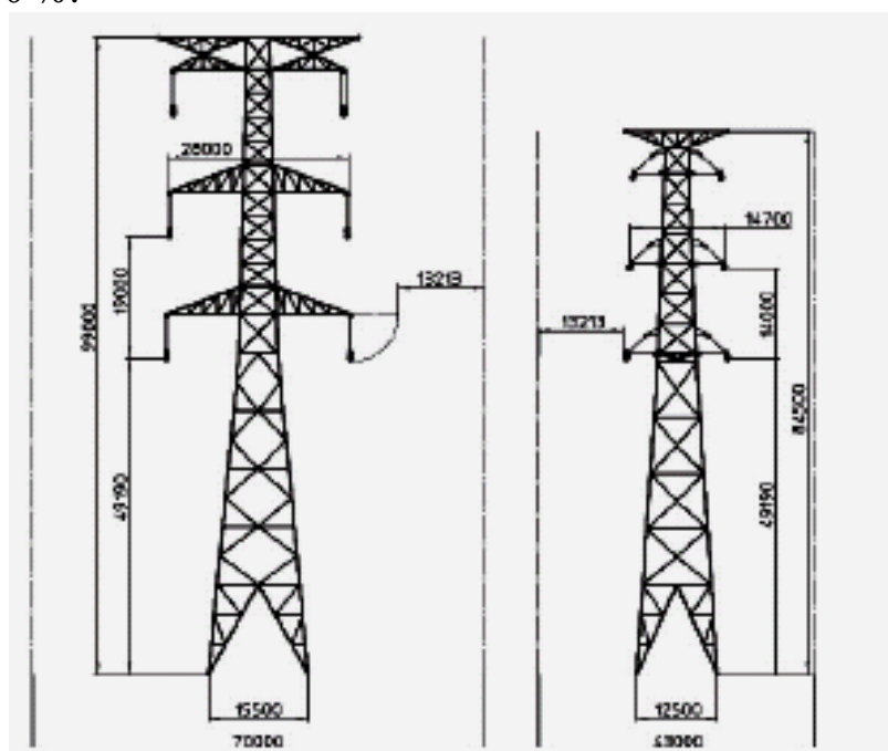
Рис.4. Конфигурация и размеры обычной двухцепной ВЛ и компактной линии 765 кВ с V-образными изолирующими траверсами
