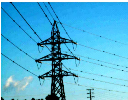
Рис.6. Устройства повышения визуальной доступности проводов ВЛ
